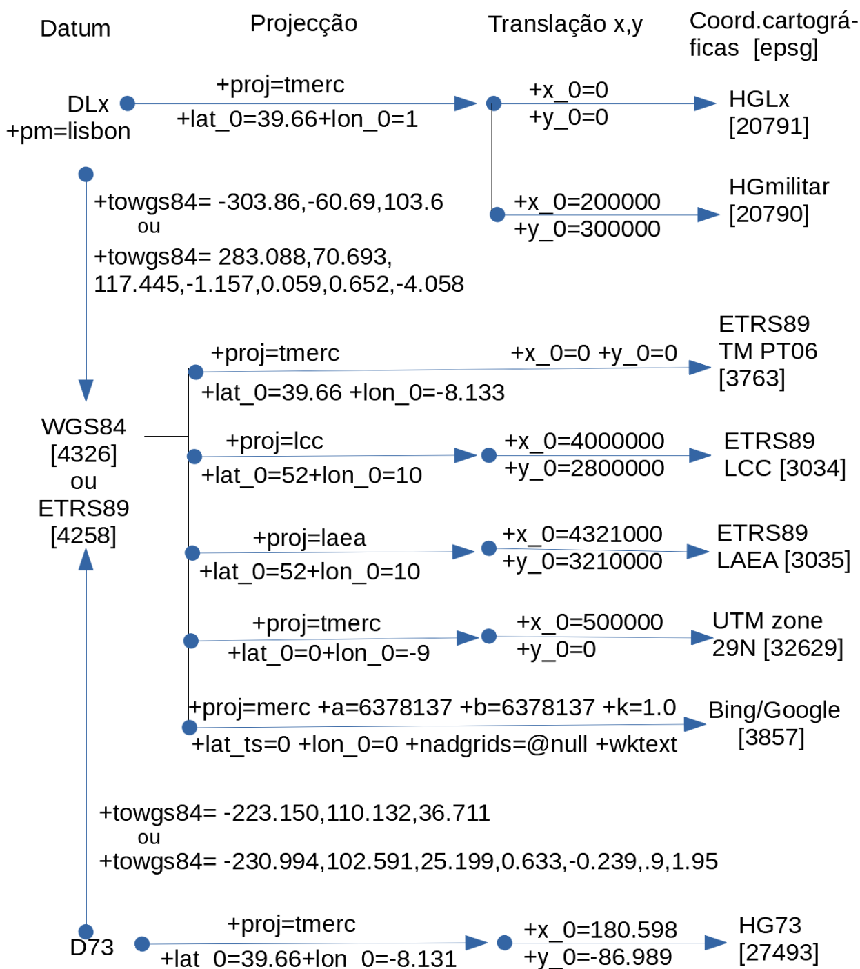
Figura 20. Algumas tranformações de datum, projecções e translações de coordenadas úteis para a cartografia de Portugal Continental para reprojectar um sistema de coordenadas de referência num outro (nem todos os parâmetros proj4 estão indicados e alguns parâmetros estão truncados – ver Tabela 2)
