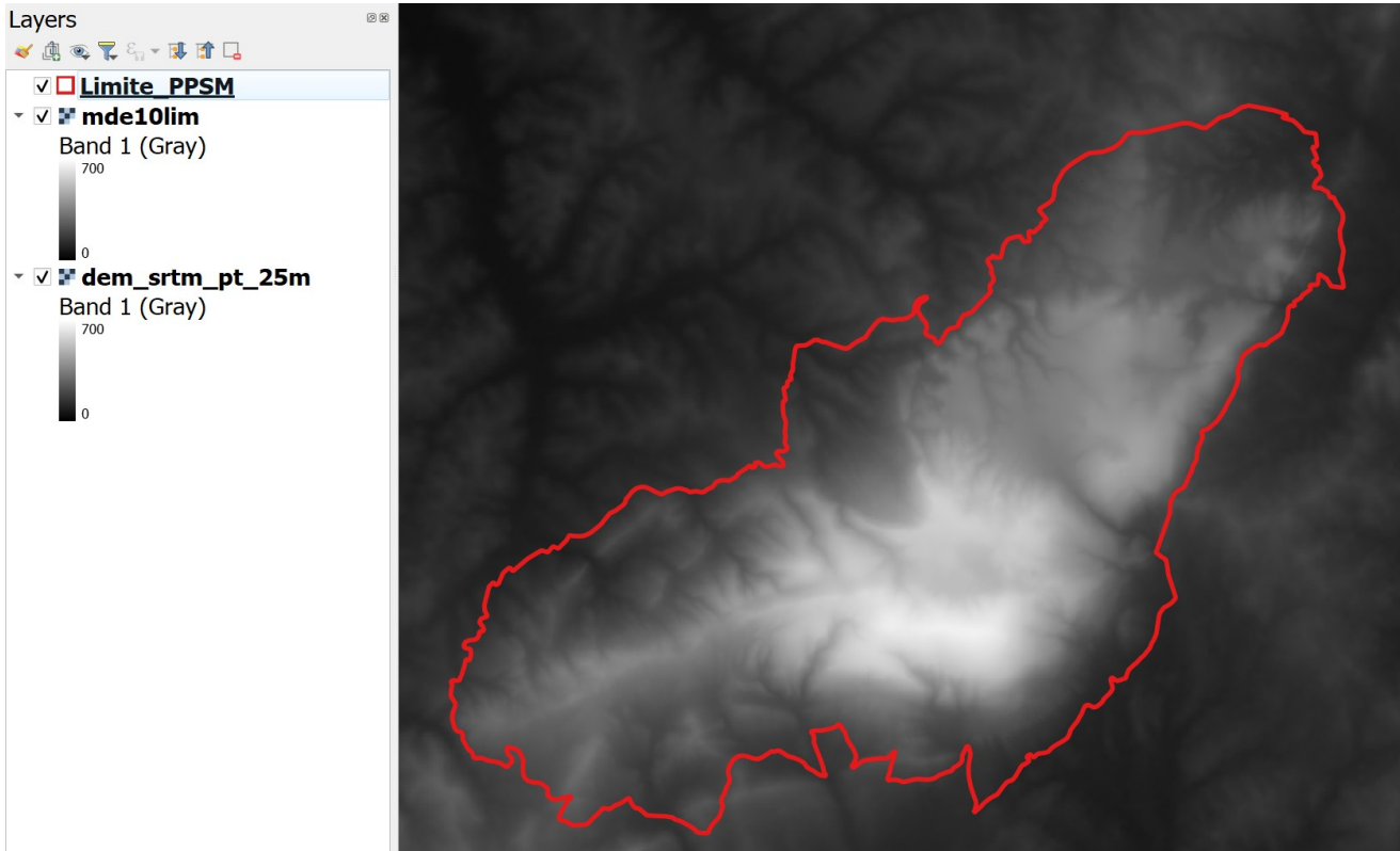
Figura 23. Comparação de MDE SRTM reamostrado a 25 m na região da Paisagem Protegida da Serra de Montejunto com o MDE derivado de dados topográficos com interpolação TIN e resolução espacial de 10 m (por cima). É visível que a resolução espacial é mais fina no interior da PPSM.
