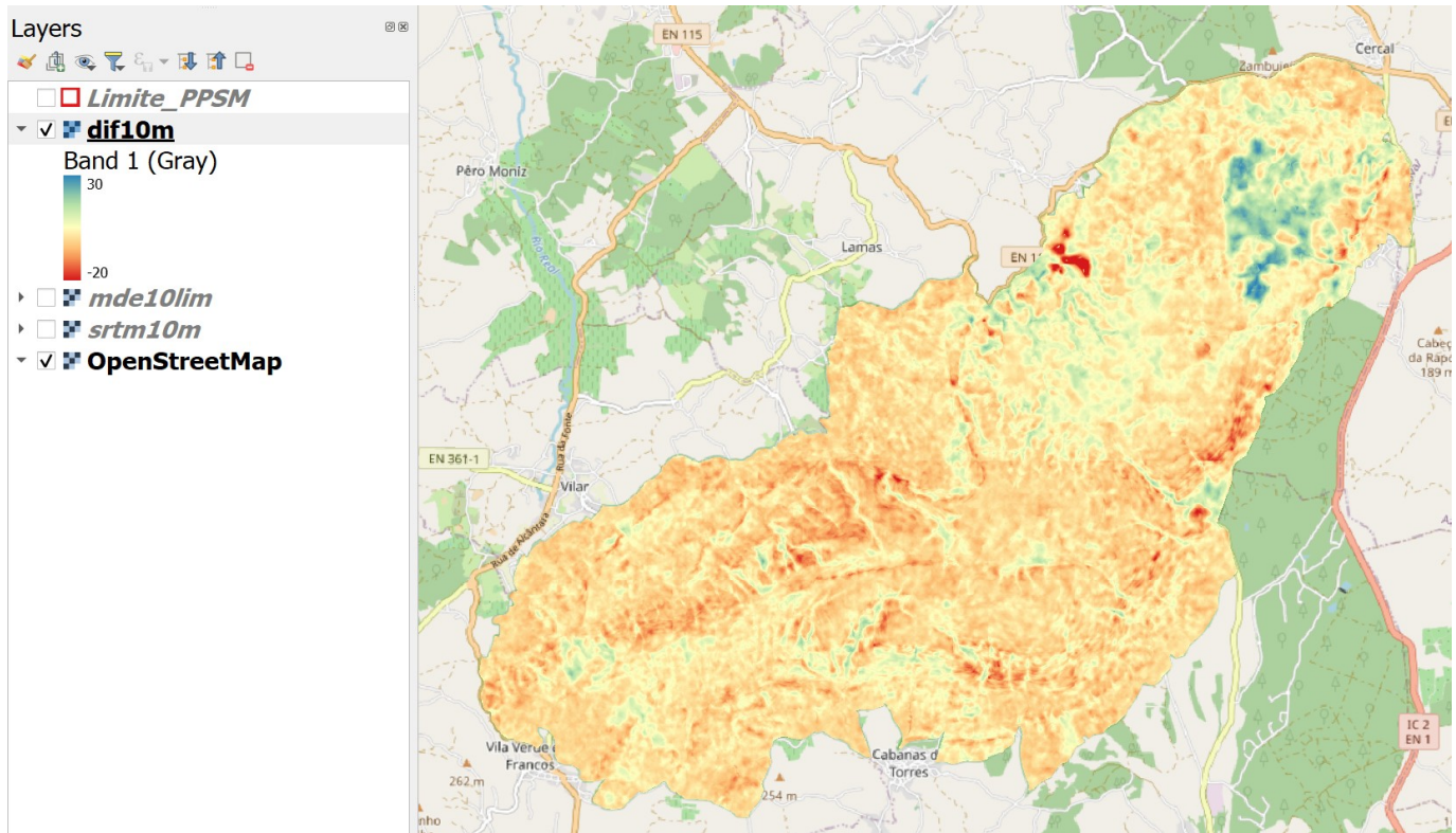
Figura 24 Paisagem Protegida da Serra de Montejunto: diferenças em metros entre a carta de elevações derivada de dados topográficos e carta de elevações derivadas de SRTM3. Os valores negativos (a vermelho) correspondem a zonas em que a elevação (dados topográficos) é inferior à elevação indicada pelos dados abertos dem_srtm_pt_25m.
