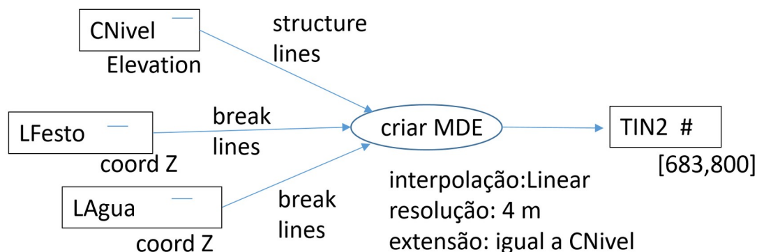
Figura 22. Diagrama de operações para descrever a construção de um MDE a partir de informação de levantamento topográfico
