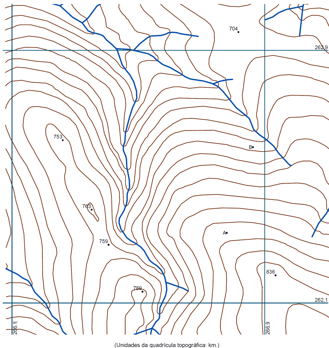
Figura 21. Carta topográfica que usa sistema de coordenadas de referência EPSG: 20790 (“coordenadas militares”)
