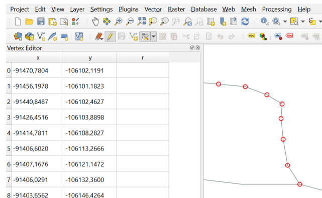
Figura 4: Painel “vertex editor” e representação geométrica dos pontos respectivos em QGIS 3
