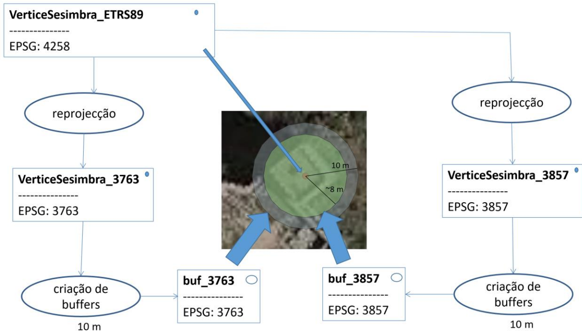
Figura 18. Diagrama de operações para calcular buffer em torno do ponto VerticeSesimbra em dois sistemas de coordenadas de referência distintos, um com distorções muito pequenas (epsg:3763) e outro com grandes distorções nas distâncias entre pontos (epsg:3857).
