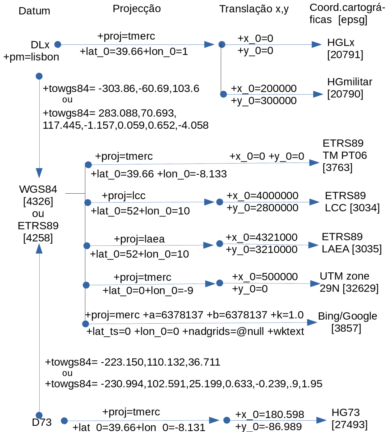
Figura 20. Algumas transformações de datum, projecções e translações de coordenadas úteis para a cartografia de Portugal Continental para reprojectar um sistema de coordenadas de referência num outro (nem todos os parâmetros proj4 estão indicados e alguns parâmetros estão truncados – ver Tabela 2)
