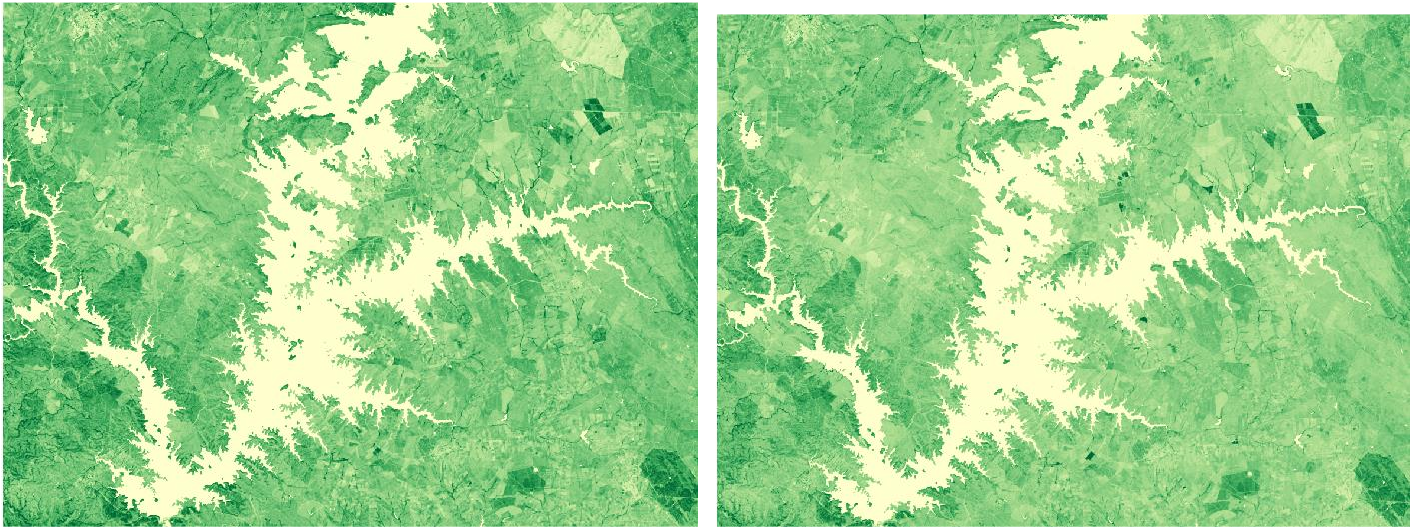
Figura 26: Carta de NDVI para dia 31 de maio (à esquerda) e para dia 15 de junho 2014 (à direita) sobre a região do Alqueva. A cor verde representa valores de NDVI mais elevados.
